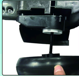
Setzen Sie die Achse in die untere Nut des Gehäuses ein
