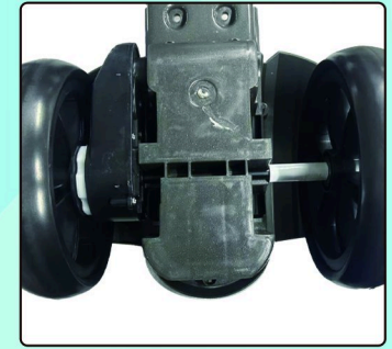
Montiertes Rad
