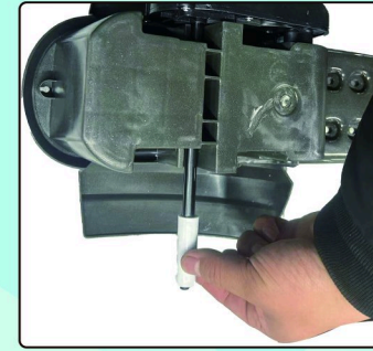
Montage der Kunststoffteile
