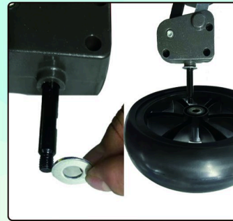
Die Dichtung aufsetzen Das Rad an der Achse befestigen
