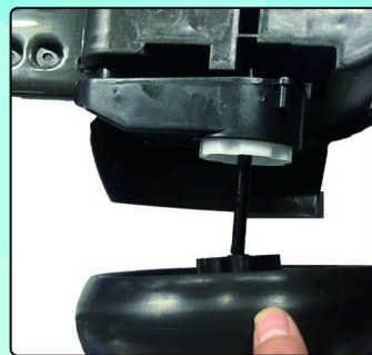
Umetnite osovinu u donji žlijeb kućišta
