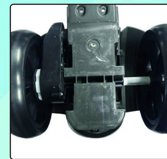
Namontované kolo
